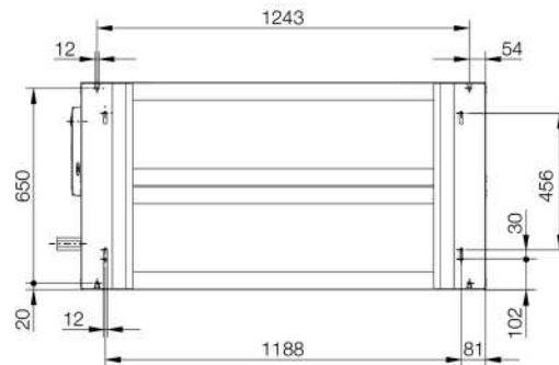
Ansicht von unten / bottom view / vue de dessous
